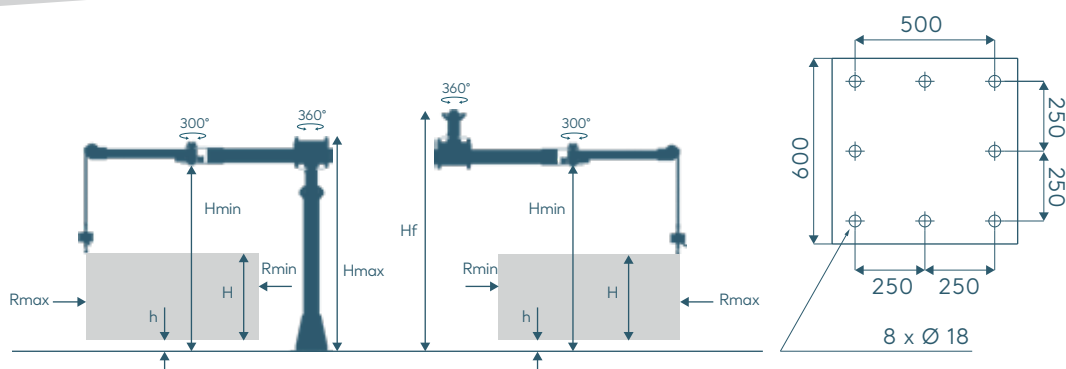
Fußplattenmaße [mm]
